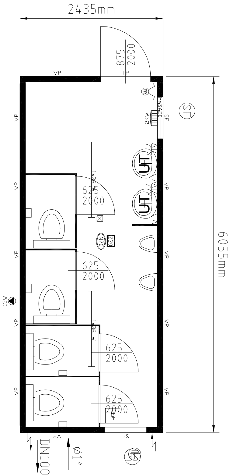
203186.dwg
