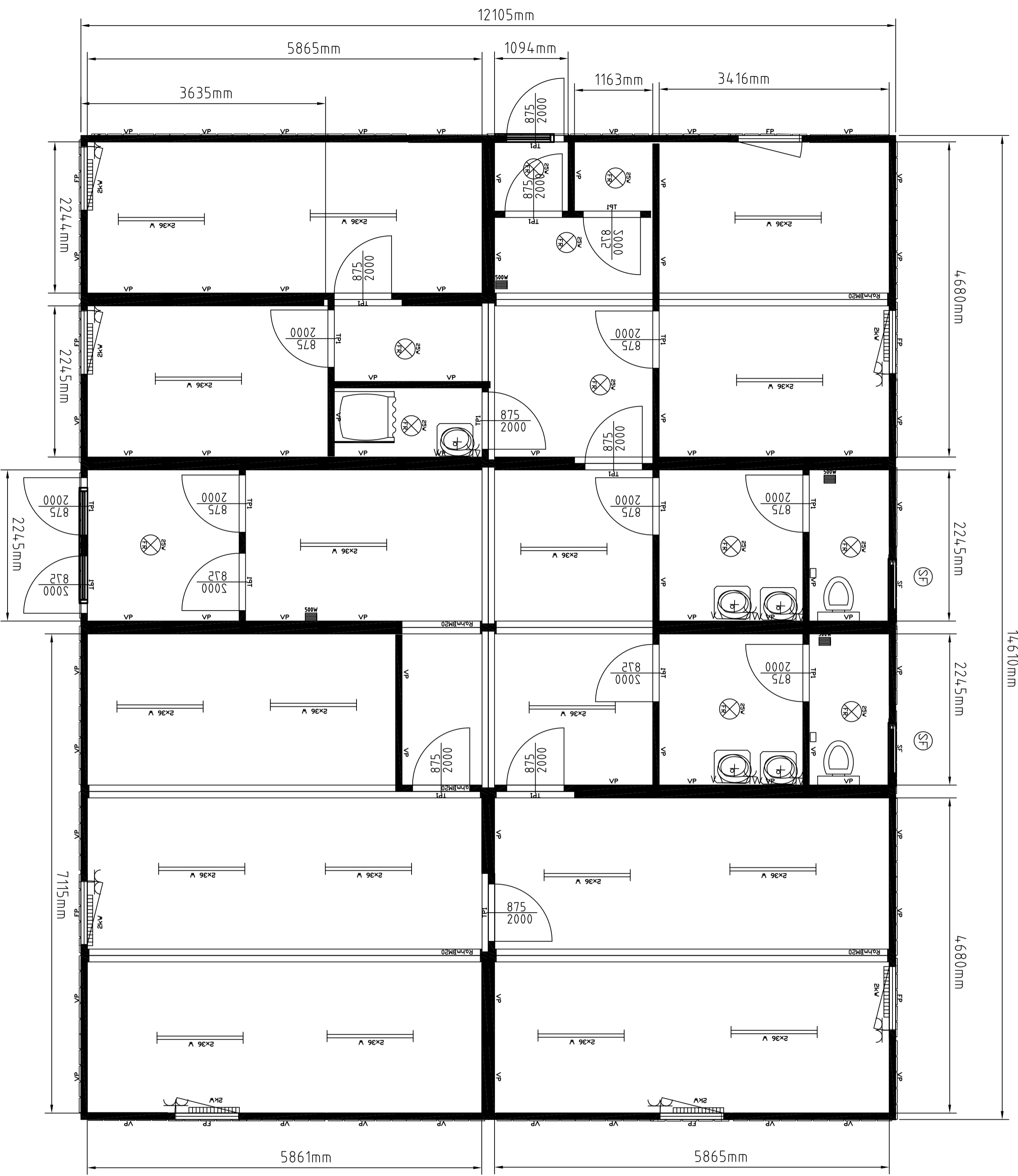
Сельская школа.dwg
